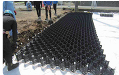
ジオセル展開2
